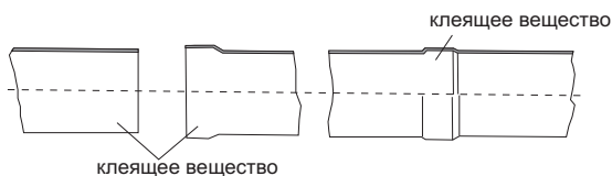
Рисунок 18 – Простое соединение жесткого типа, путем склеивания
