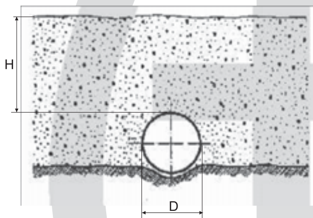
Рисунок 11 – Укладка в укрепительном сооружении (положительное расположение)
