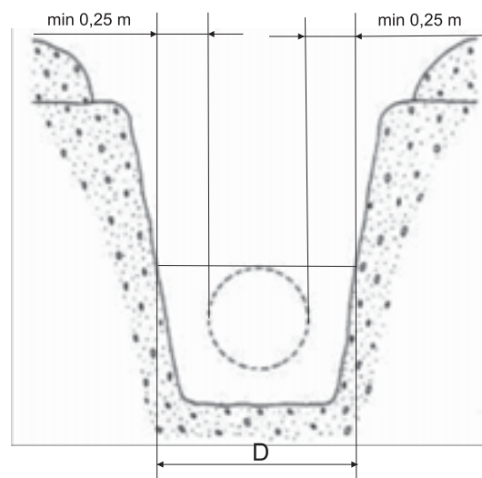
Рисунок 14 – Ширина канавы
