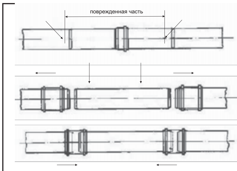
Рисунок 30 Ремонт трубопровода
