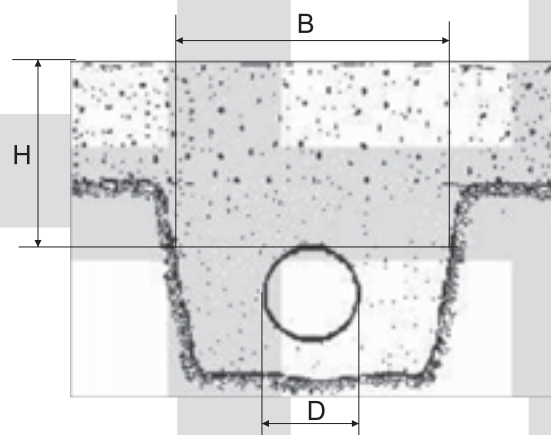
Рисунок 12 – Укладка в укрепительном сооружении (отрицательное расположение)
