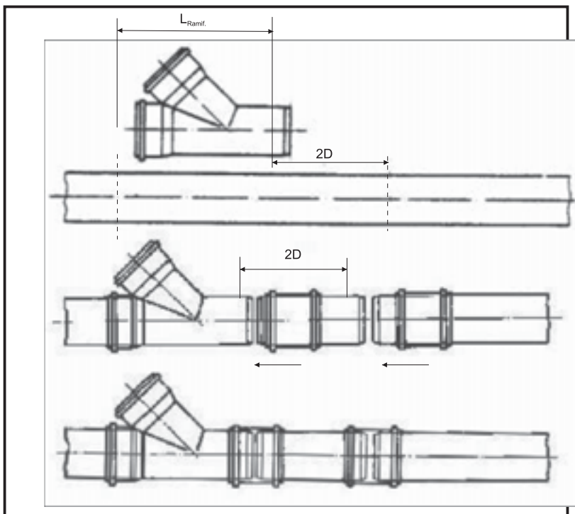
Рисунок 31 Использование разводов и двух разъемных раструбов
