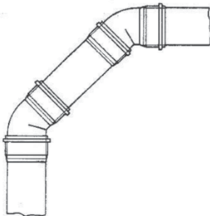
Рисунок 23 Изгиб под углом 90^\circ со вставкой трубы
