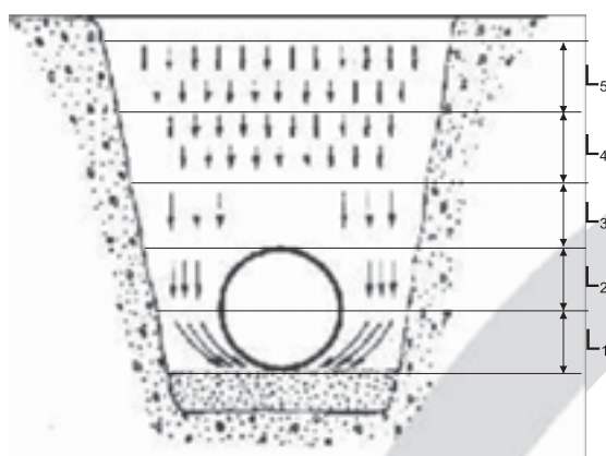
Рисунок 16 Последовательное заполнение канавы слоями
