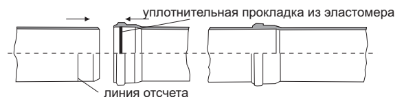
Рисунок 21 – Соединение с раструбом, эластичного типа, с уплотнительной прокладкой (эластомер)
