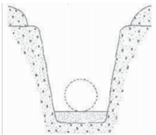
Рисунок 15 – Фундаментный слой
