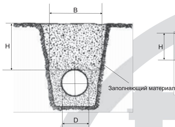
Рисунок 9 – Узкая канава
