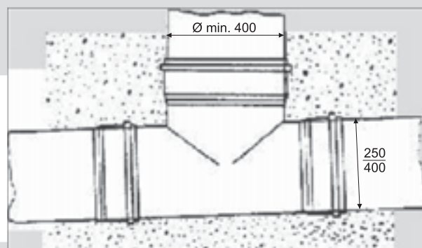
Рисунок 29 Линейный колодец из пластика
