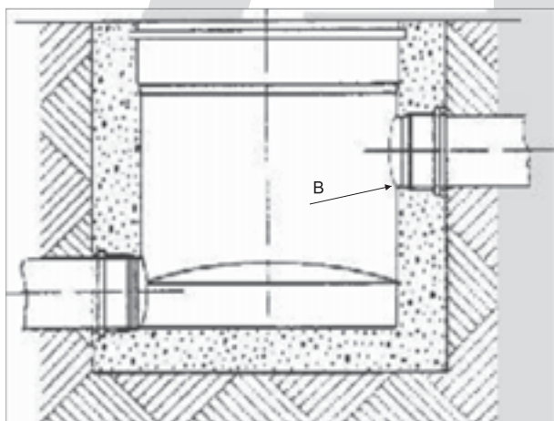
Рисунок 28 Колодец с перепадом в диаметре, со сплошным материалом
