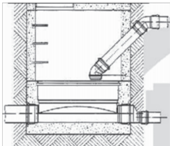
Рисунок 26 Линейный колодец с соединениями и перепадом в диаметре основного трубопровода
