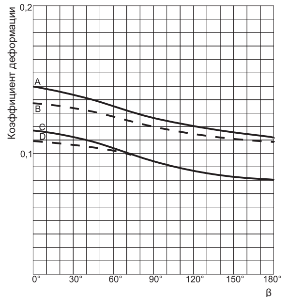
Рисунок 8 Коэффициент деформации трубы под нагрузкой
