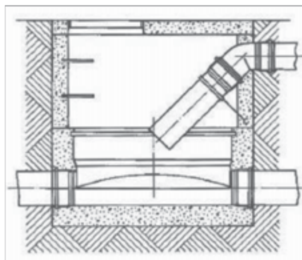
Рисунок 25 Линейный колодец с вводом для нужд абонентов
