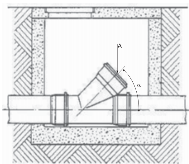
Рисунок 26 Колодец для осмотра и очистки
