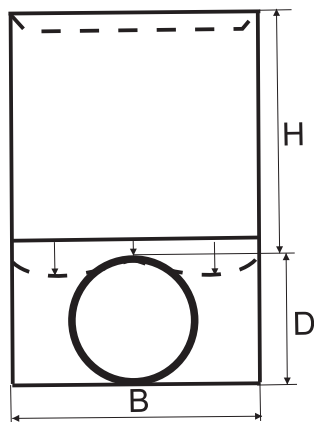
Рисунок 3 Осадка грунта для жесткой трубы
