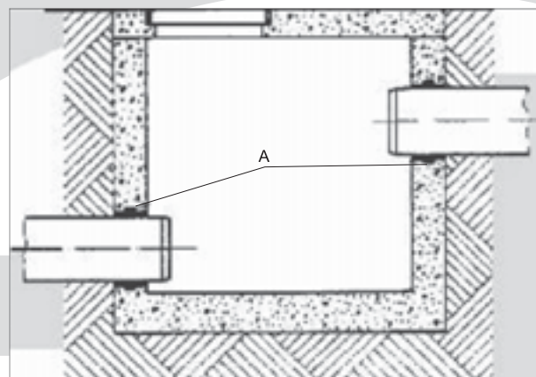
Рисунок 27 Колодец без неразрывности материала
