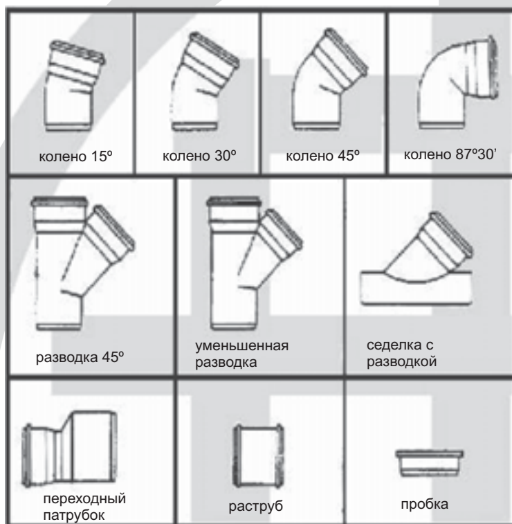
Рисунок 22 Специальные фитинги и детали, наиболее часто используемые
