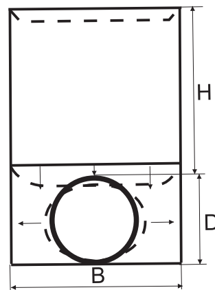
Рисунок 4 Осадка грунта для гибкой трубы
