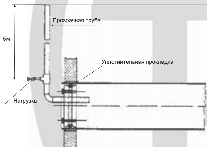
Рисунок 38 Пример закрытия для испытания гидравлической герметичности
