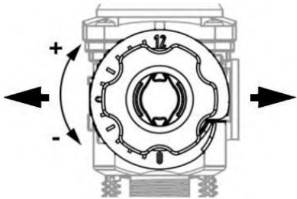
Мал. 14. Регуляційна ручка пластикового витратоміра
