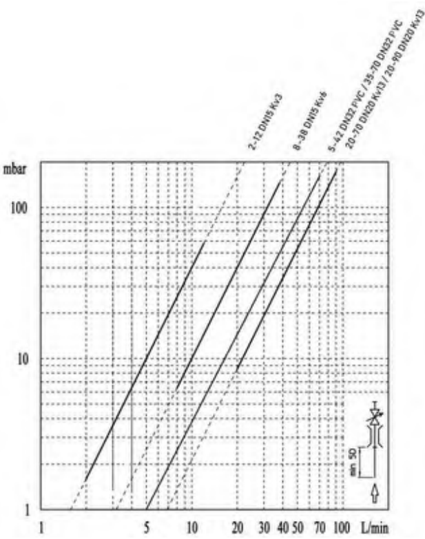
Мал. 15. Характеристика гідравлічних втрат для всіх витратомірів PRAWTECH
