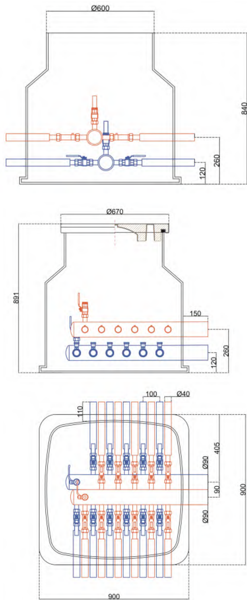
Мал. 6. Розміри та конструкційні параметри колодязя Terra MINI (11 секції)
