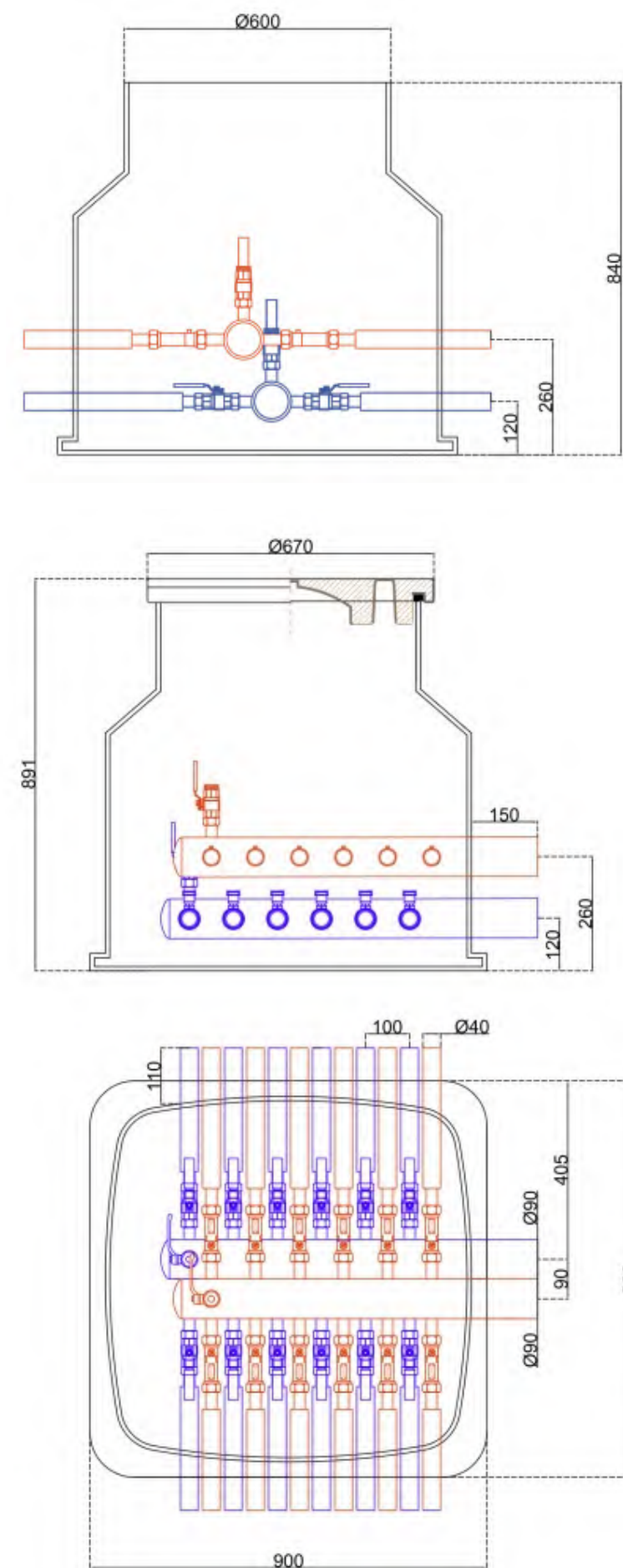
Мал. 7. Розміри та конструкційні параметри колодязя Terra MINI (12 секції)
