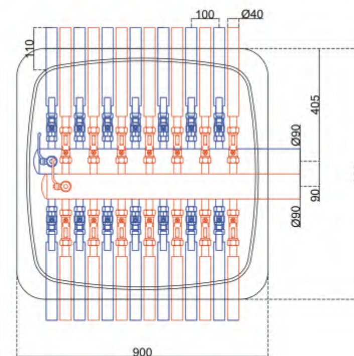
Мал. 7. Розміри та конструкційні параметри колодязя Terra MINI (14 секції)
