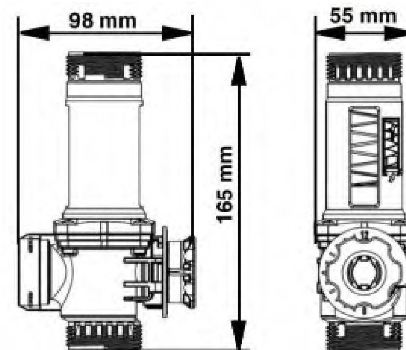
Мал. 13. Витратомір типу E: 5–42 л/хв
