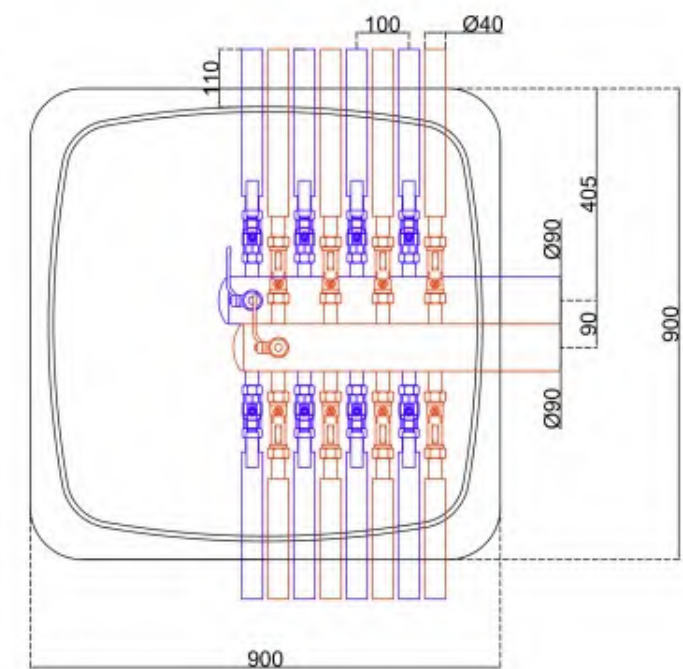
Мал. 7. Розміри та конструкційні параметри колодязя Terra MINI (8 секції)
