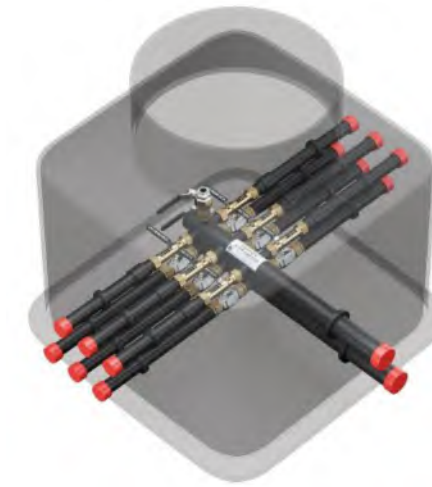
Мал. 1. Приклад внутрішньої частини колодязя Terra Opti
