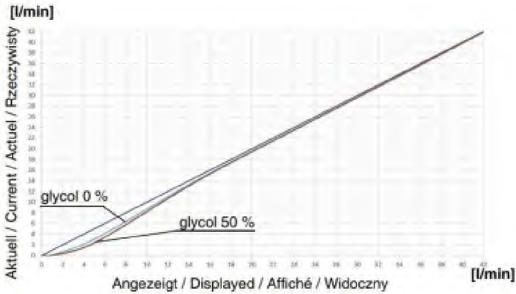
Мал. 15. Коригувальна крива для пластикових витратомірів
